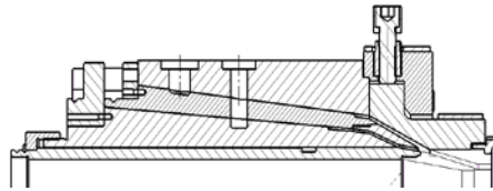
前方手動調芯
